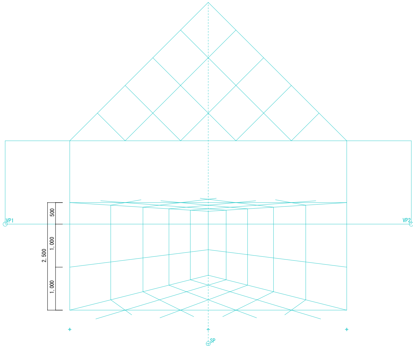
2 消点パースグリッド 910mm × 910mm × CH2,500mm (手前 1/50)
